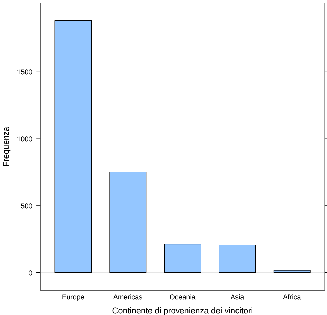
Grafico a barre w_continent
